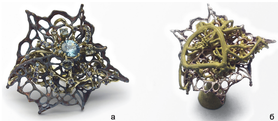
Рис. 3. а – каблучка “Hybrid casting #3: Two rivers”. Патинована мідь, золото жовтого кольору, дорогоцінне каміння. Подвійне литво. Сираurium; б – необроблена частина каблучки після подвійного литва. Сираurium
