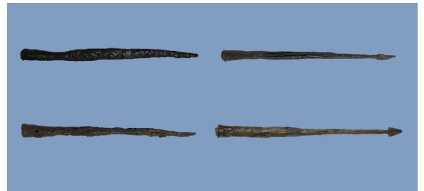
Рис. 4. Залізні наконечники дротиків та наконечник списа зі скіфського кургану № 11 с. Львово Херсонської обл. (після реставрації).
